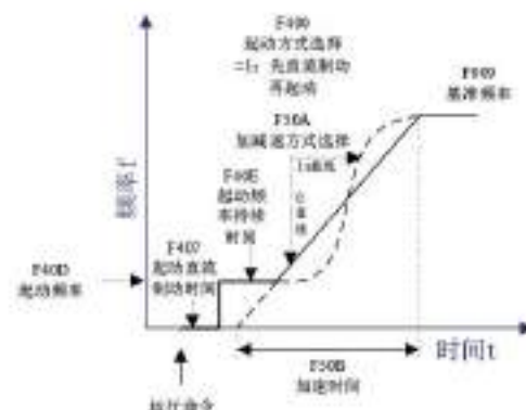
图 5-4 先直流制动再启动
