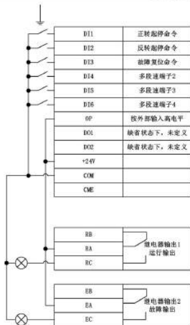
图 7-1 起重平移 4 档应用宏端子接线图
