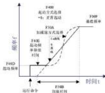
图 5-3 正常启动
