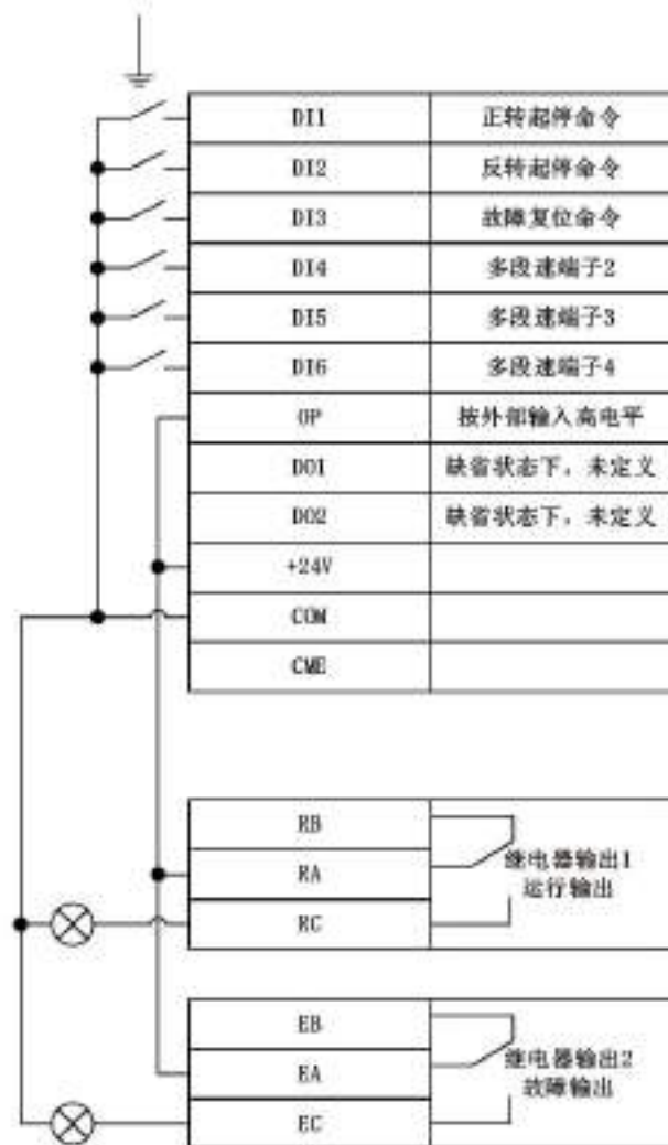
图 7-3 提升宏端子接线图
