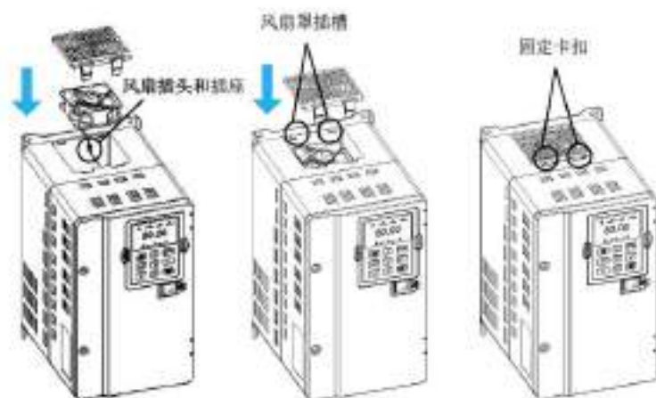
图 12-4 B~C 尺寸机型风扇安装
