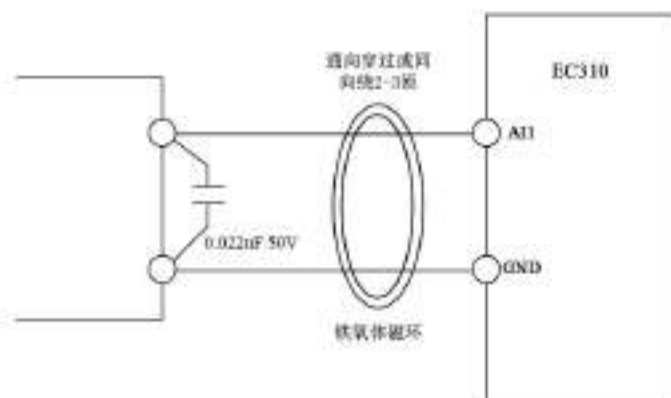
图 3-31 电流信号输入模拟量端子接线图
