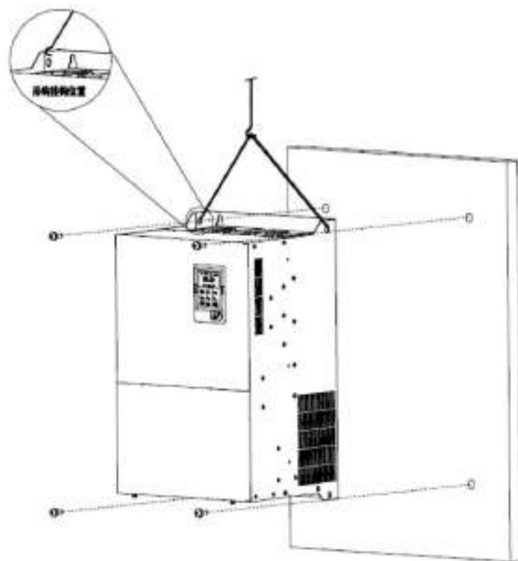
图 3-8 D~G 尺寸机型壁挂式安装示意图
