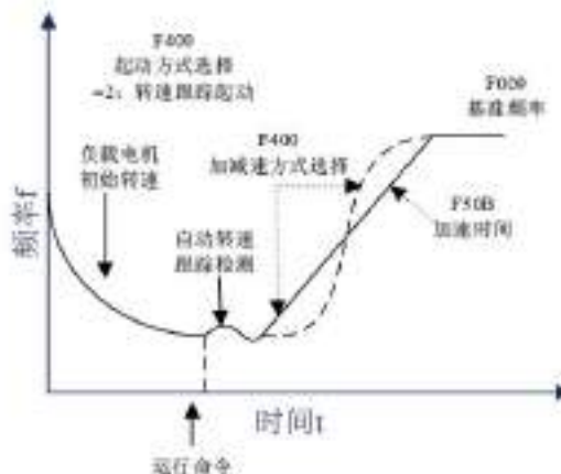
图 5-5 转速跟踪启动
