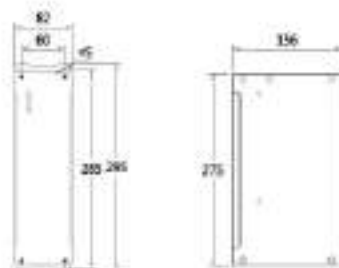
图 13-19 EC500Z-B01/B02/B03 制动单元外形尺寸图
