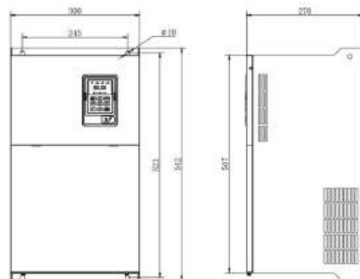
图 13-6 规格 F (45 ~ 55kW) 机型外形尺寸
