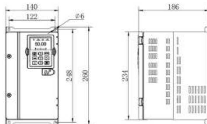
图 13-3 规格 C (7.5 ~ 11kW) 机型外形尺寸
