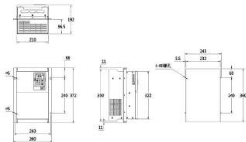
图 13-8 规格 D 机型中部安装支架及开孔尺寸
