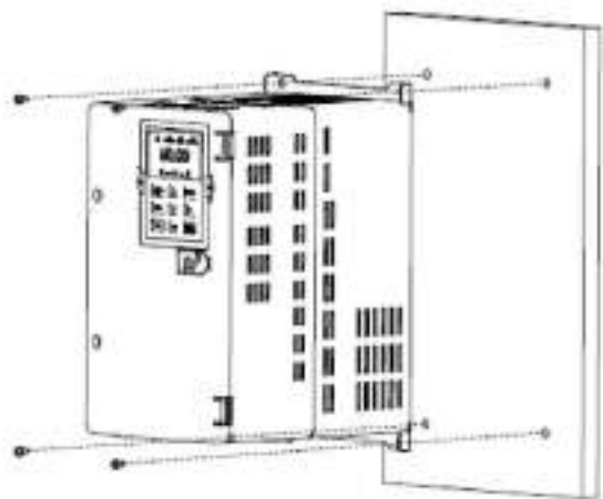
图 3-7 D~C 尺寸机型壁挂式安装示意图
