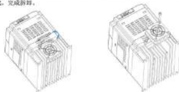
图 12-1 A 尺寸机型风扇拆卸
