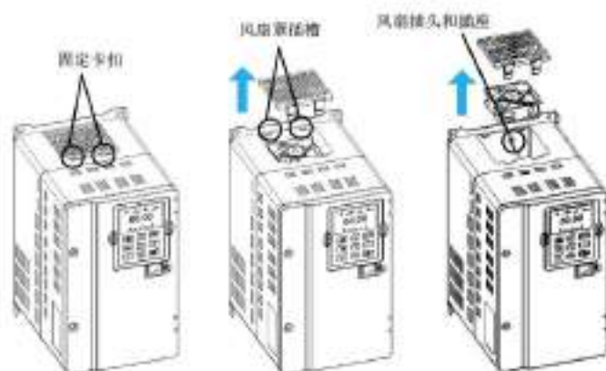
图 12-3 B~C 尺寸机型风扇拆卸
