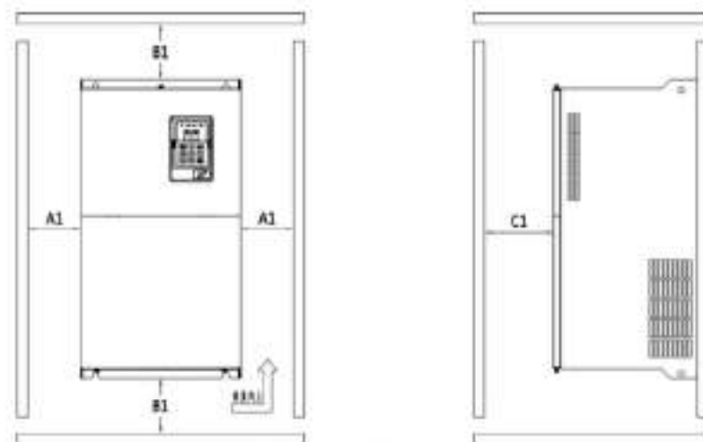
图 3-2 A~G 尺寸单机安装空间
