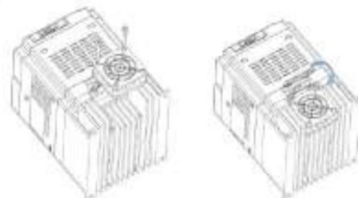
图 12-2 A 尺寸机型风扇拆卸
