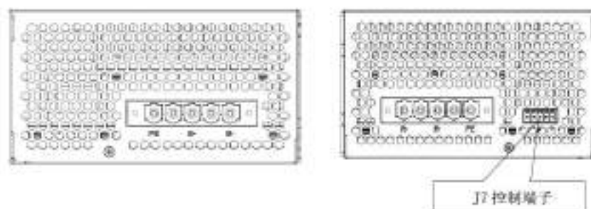
图 13-16 EC500Z-B01/B02/B03 制动单元端子分布图
