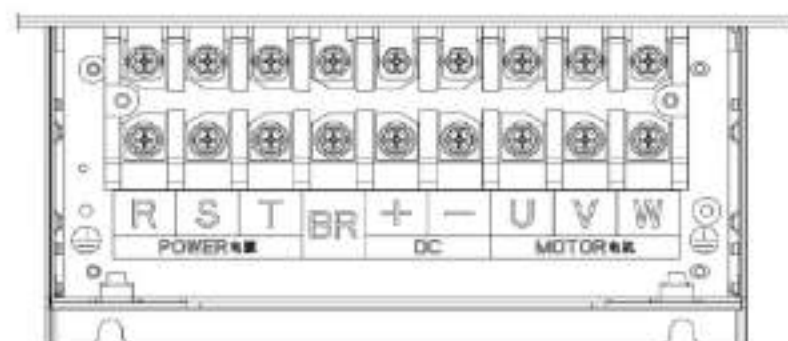
图 3-26 尺寸 B~G 机型主回路端子示意图
