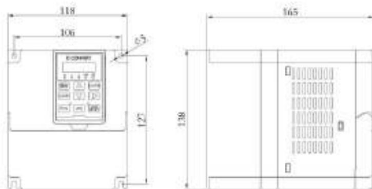
图 13-1 规格 A (0.4 ~ 3.7kW) 机型外形尺寸
