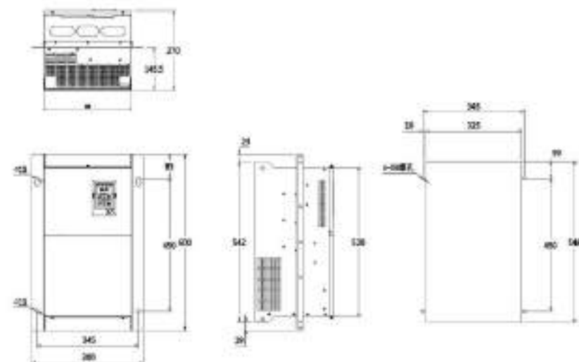
图 13-10 规格 F 机型中部安装支架及开孔尺寸
