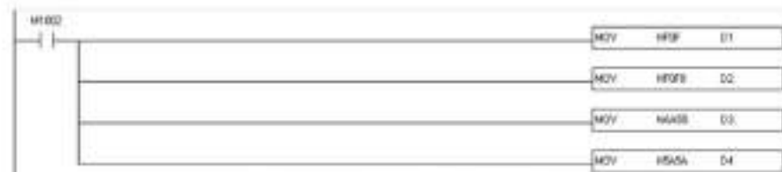
图 9-2 PLC Modbus 主站通讯设置
