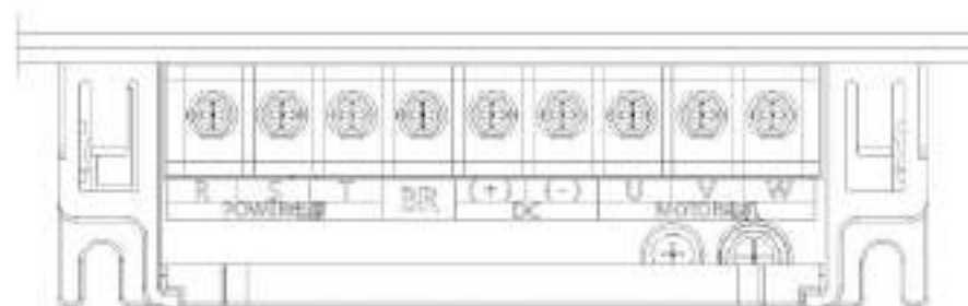
图 3-25 尺寸 A 机型主回路端子示意图
