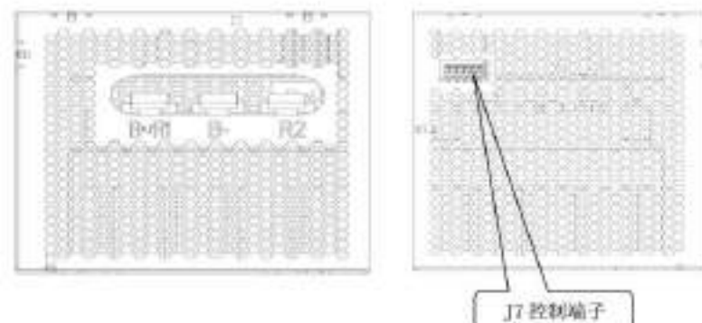
图 13-17 EC500Z-B04 制动单元端子分布图
