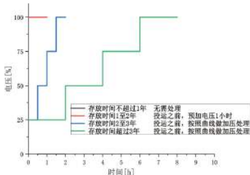
图 3-1 长期存放后投运前变频器的处理
