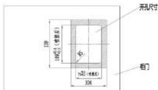
图 3-21 柜门键盘安装开孔尺寸图
