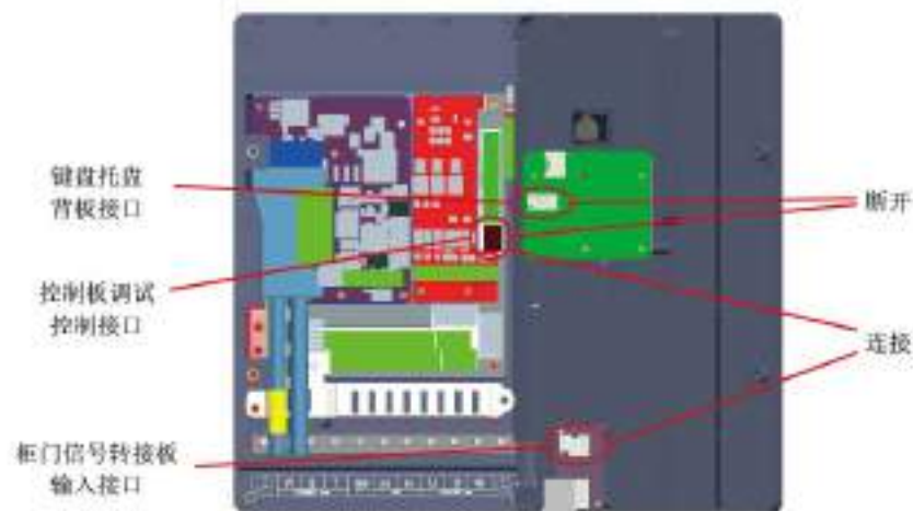
图 3-20 柜门信号转接板连接方式
