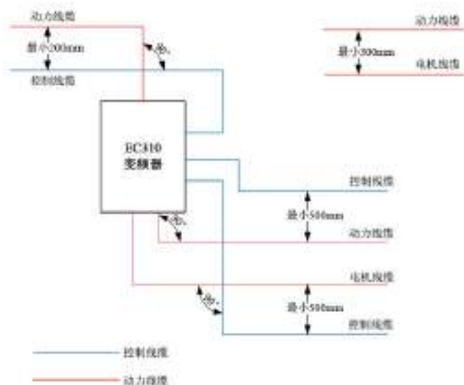
图 3-29 电缆布线图
