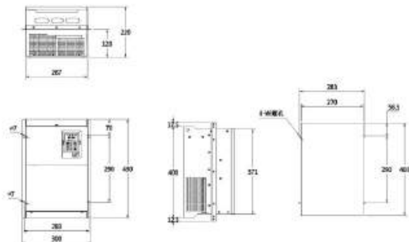
图 13-9 规格 E 机型中部安装支架及开孔尺寸
