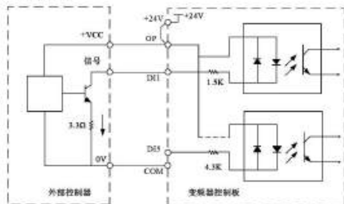
图 3-32 数字输入漏型接线方式
