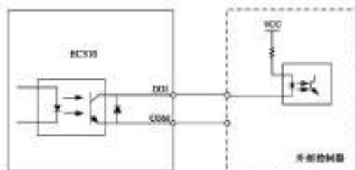
图 3-37 高速数字输出端子接线示意图
