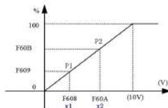
图 5-2 模拟量输入曲线
