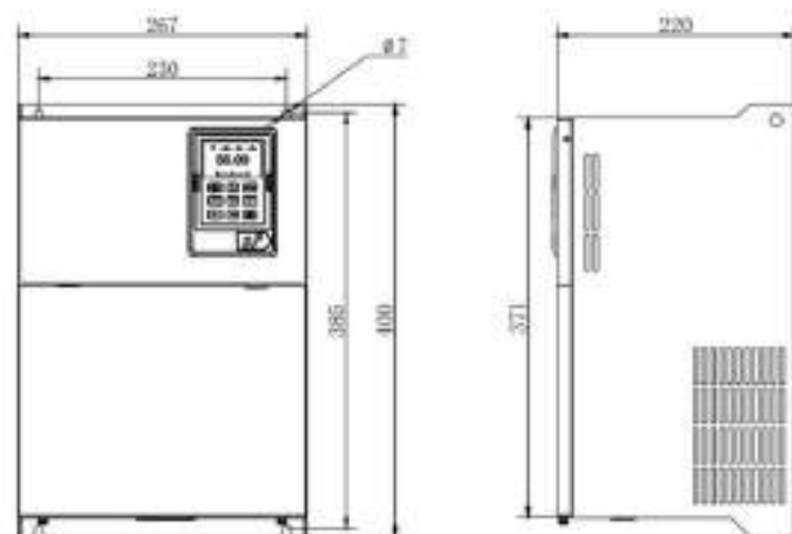
图 13-5 规格 E (30 ~ 37kW) 机型外形尺寸
