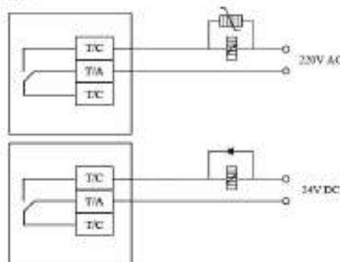
图 3-38 继电器输出端子抗干扰处理
