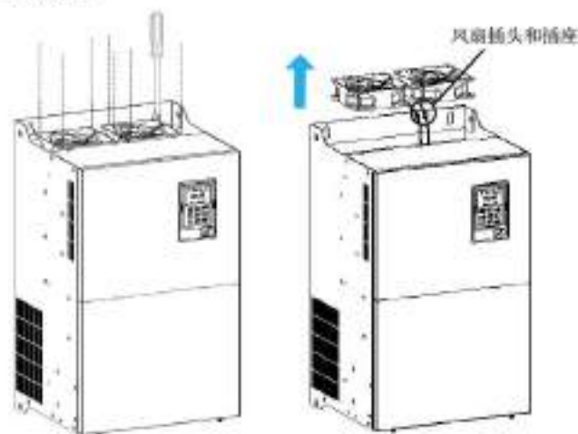
图 12-5 D~G 尺寸机型风扇拆卸
