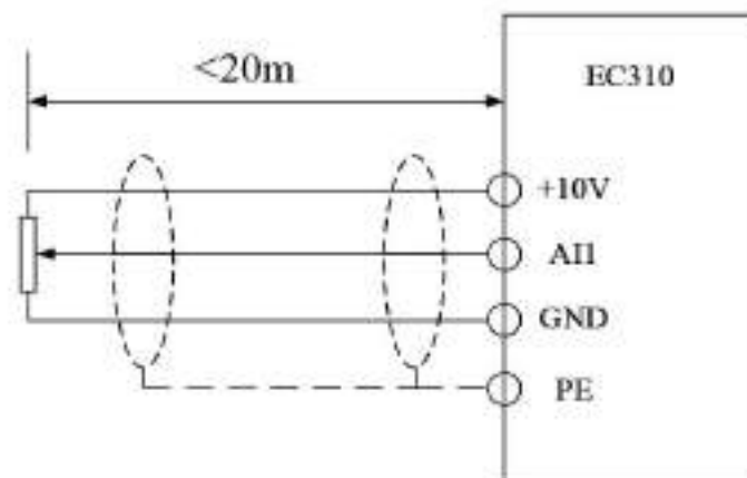
图 3-30 电压信号输入模拟量端子接线图
