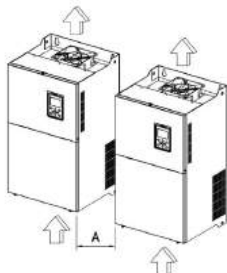
图 3-3 左右并机安装示意图
