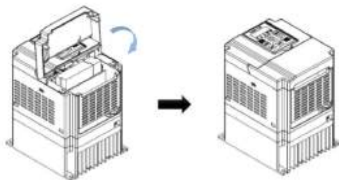
图 3-10 A 尺寸机型盖板安装示意图
