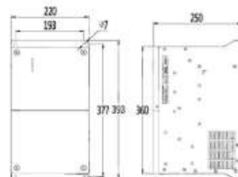
图 13-21 EC500Z-B05/B06 制动单元外形尺寸图
