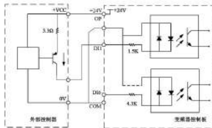
图 3-34 数字输入源型接线方式
