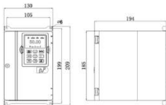
图 13-2 规格 B (5.5kW) 机型外形尺寸
