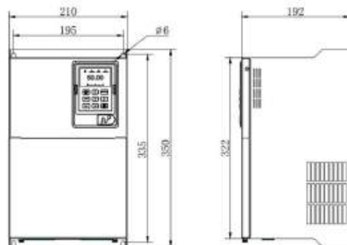
图 13-4 规格 D (15 ~ 22kW) 机型外形尺寸
