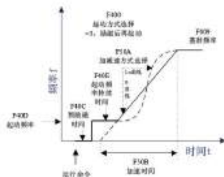
图 5-6 励磁后再启动
