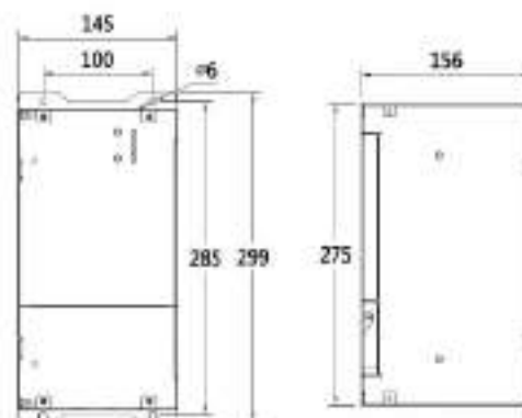
图 13-20 EC500Z-B04 制动单元外形尺寸图
