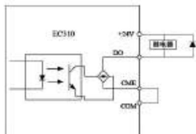
图 3-36 数字输出端子接线示意图
