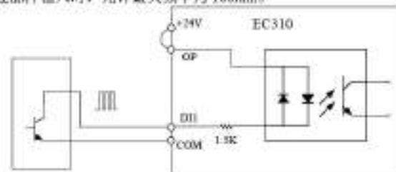
图 3-35 高速脉冲输入
