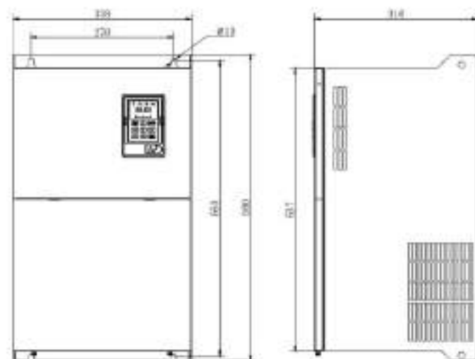
图 13-7 规格 G (75 ~ 110kW) 机型外形尺寸
