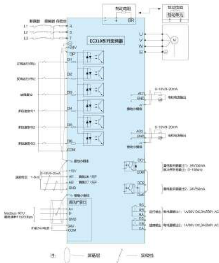
图 3-24 EC310 系列变频器典型接线图
