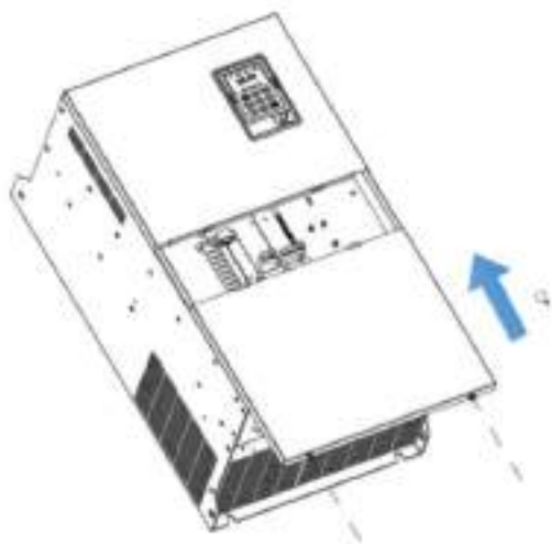
图 3-14 D~G 尺寸机型盖板安装示意图
