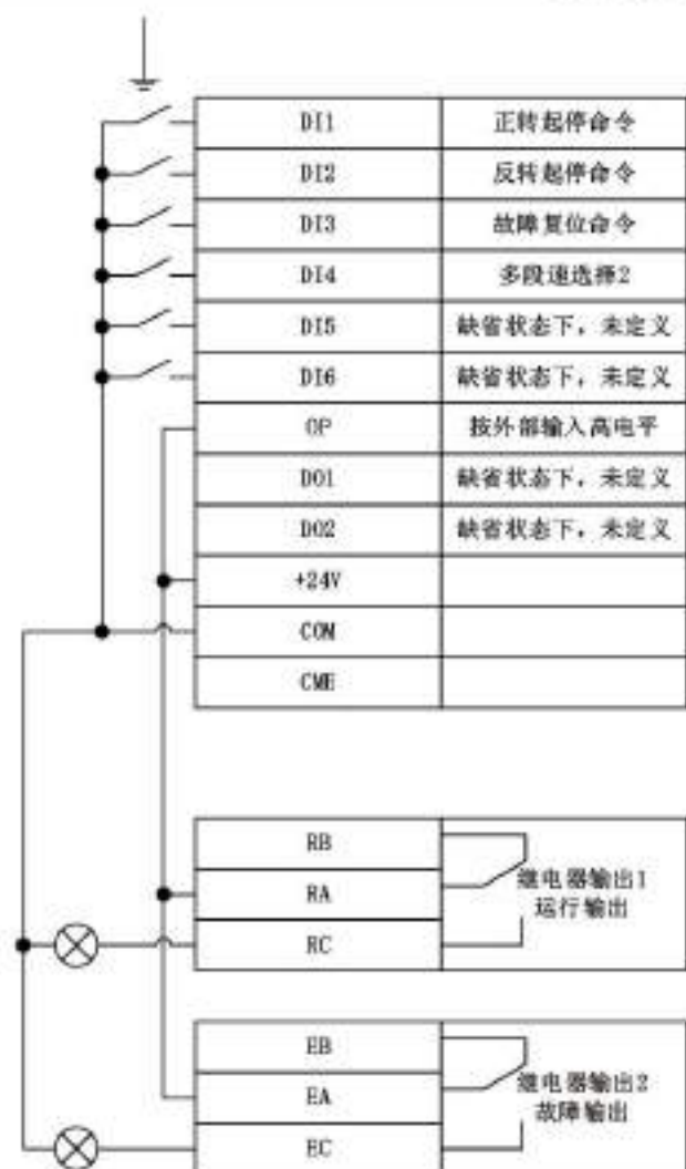
图 7-4 起重平移 2 档应用宏端子接线图
