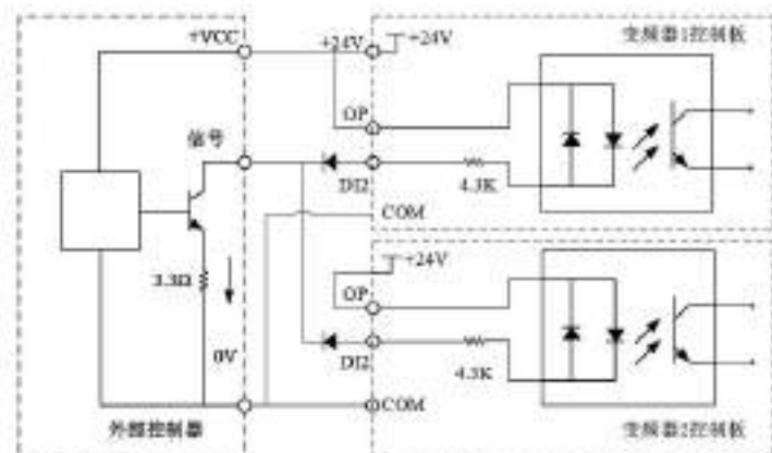
图 3-33 多台变频器 DI 端子并接漏型接线方式
