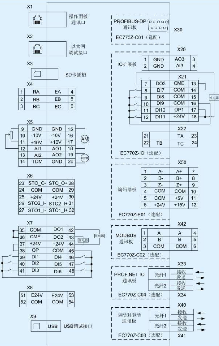
控制单元接线图
