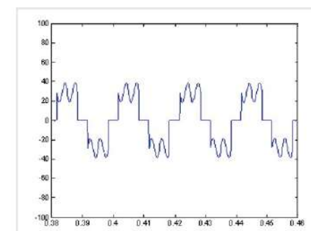
有直流电抗器：电流畸变率 35%
