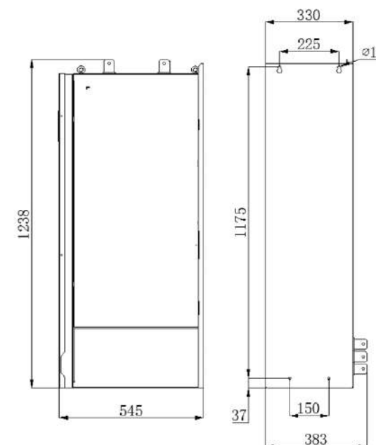
规格 J (250~280kW)
