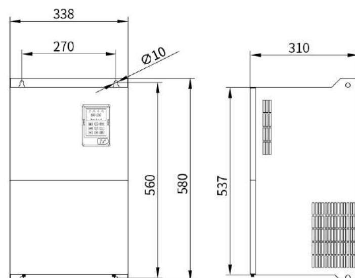
规格 G (75~110kW)
