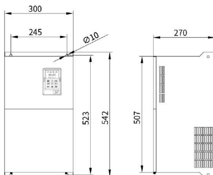
规格 F (45~55kW)
