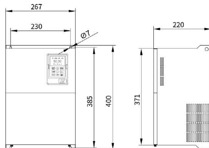
规格 E (30~37kW)
