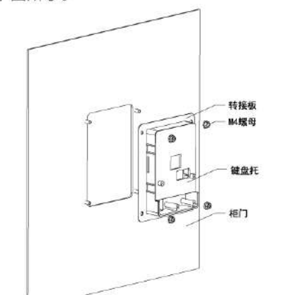
简易键盘柜门安装组件示意图 (螺丝安装)
