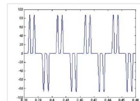
无直流电抗器：电流畸变率 90%
