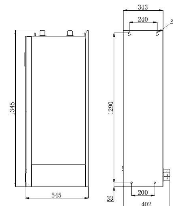
规格 K (315~355kW)
