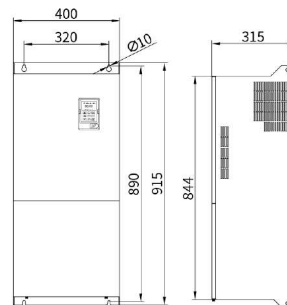
规格 H (132~160kW)
