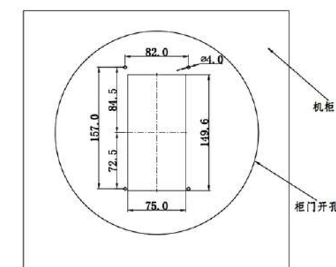
多功能键盘柜门安装组件安装开孔尺寸图
